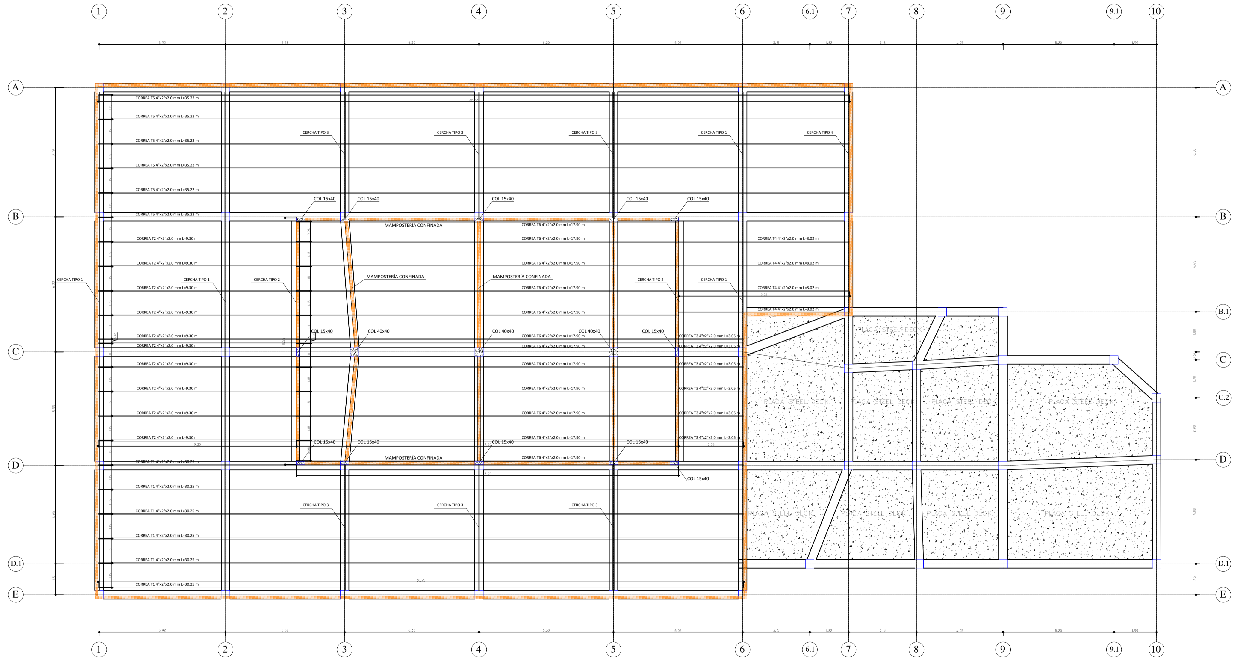
PLANTA DE CUBIERTA ESCALA 1_75
