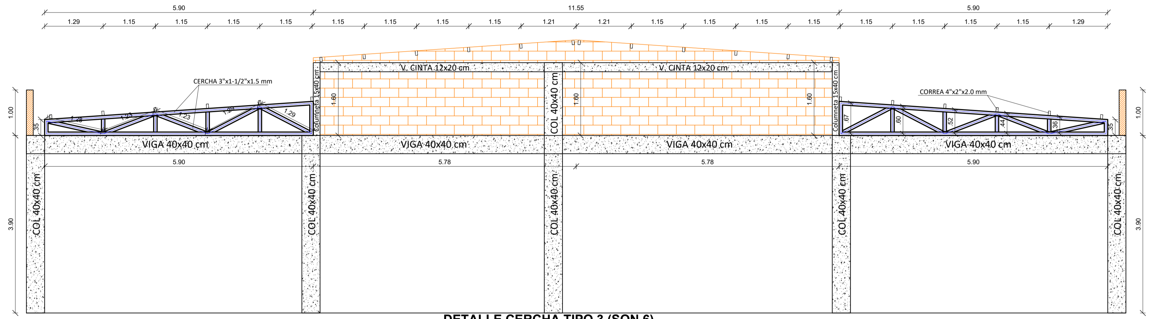
DETALLE CERCHA TIPO 3 (SON 6)
