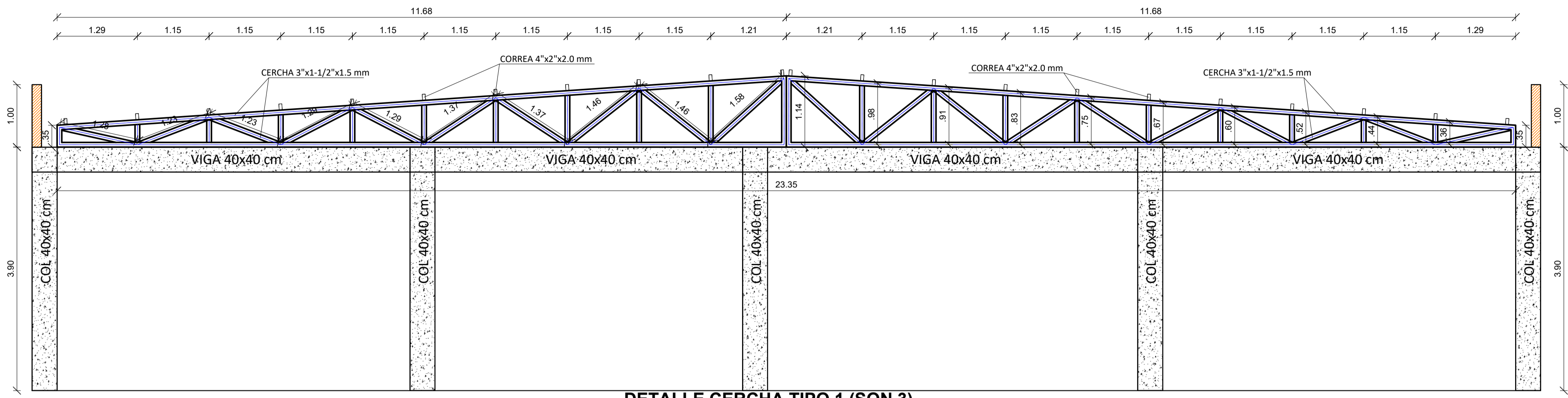
DETALLE CERCHA TIPO 1 (SON 3)
